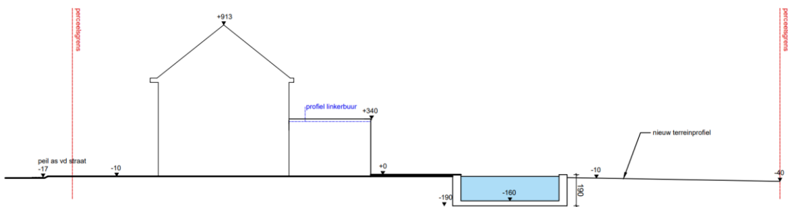
TERREINPROFIEL nieuwe toestand schaal 1/200
