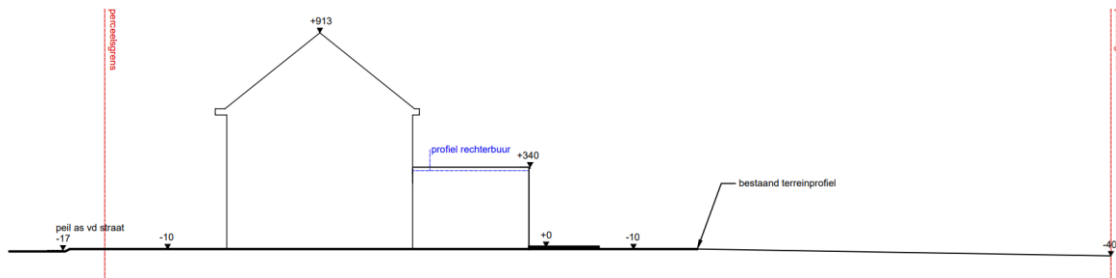
TERREINPROFIEL bestaande toestand schaal 1/200
