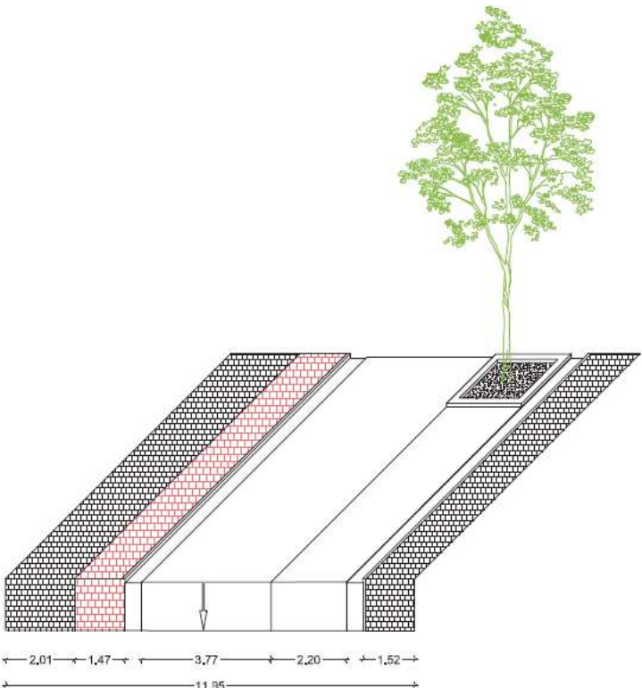
bestaand profiel
