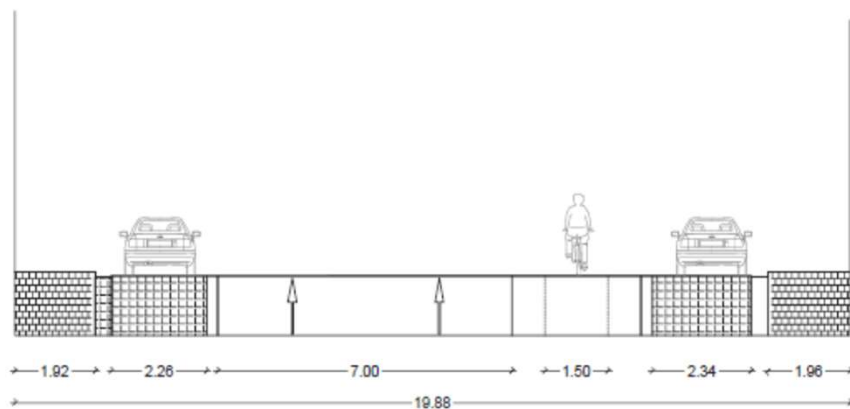
bestaand profiel
