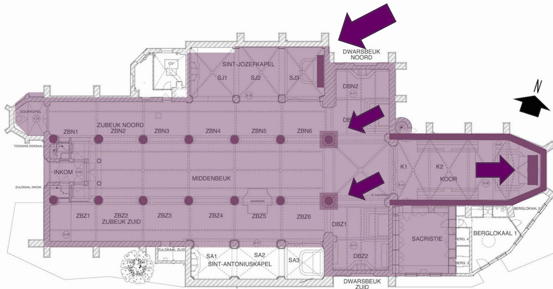
GRONDPLAN
