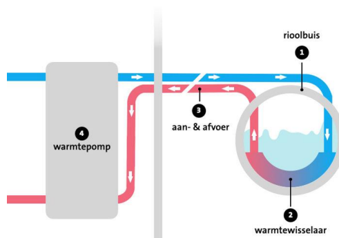
Principeschema (bron riothermie.be)
