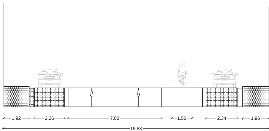
bestaand profiel
