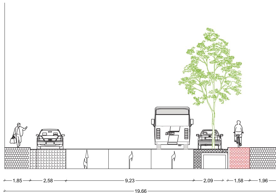
bestaand profiel
