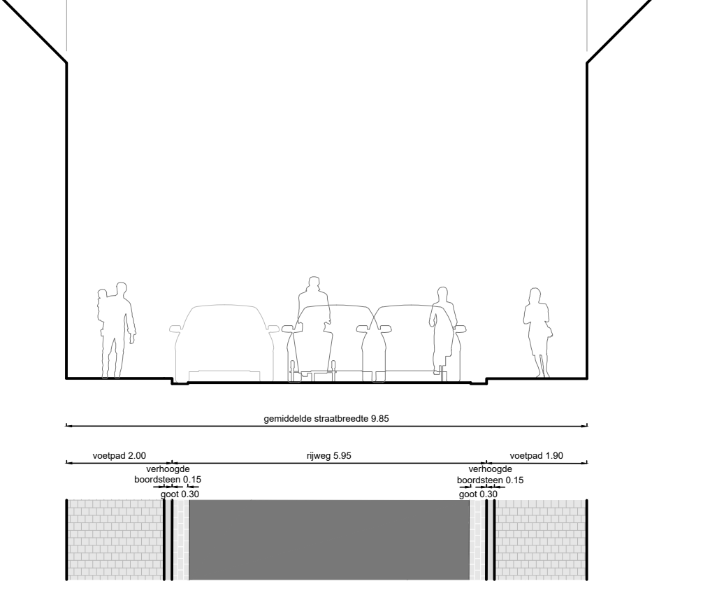
Dahliastraat typeprofiel smal - bestaand
