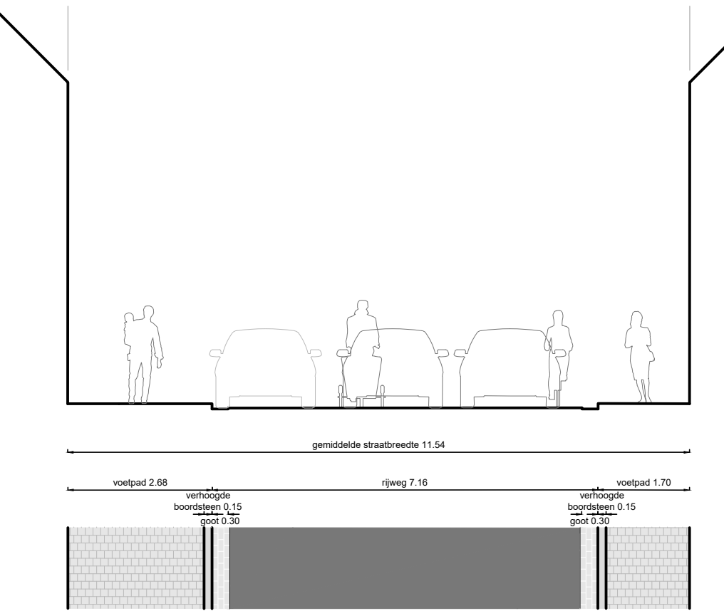
Dahliastraat typeprofiel breed - bestaand
