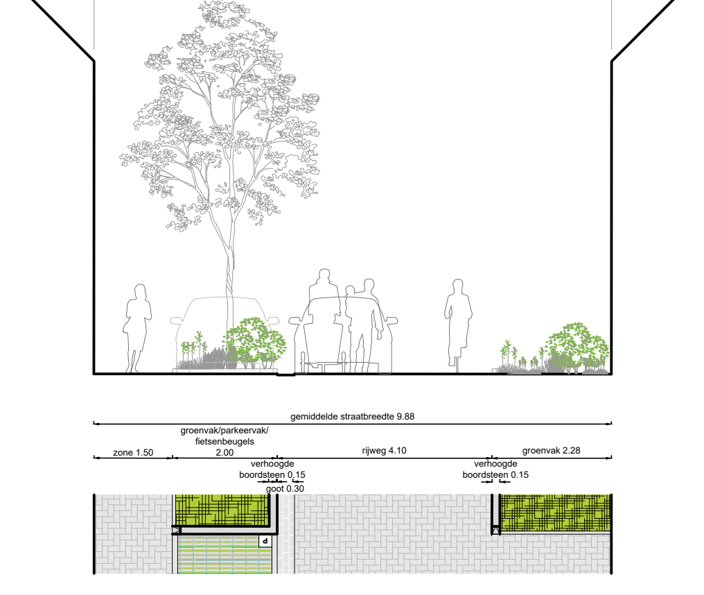
Dahliastraat typeprofiel smal - nieuw
