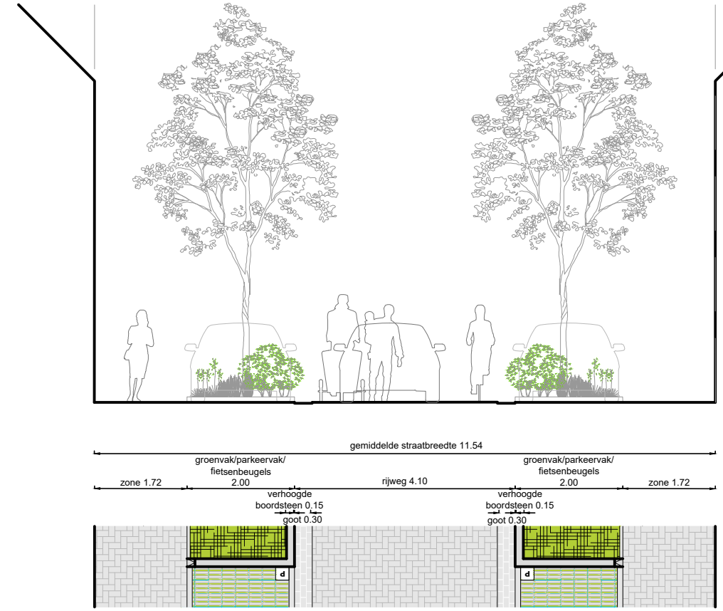
Dahliastraat typeprofiel breed - nieuw
