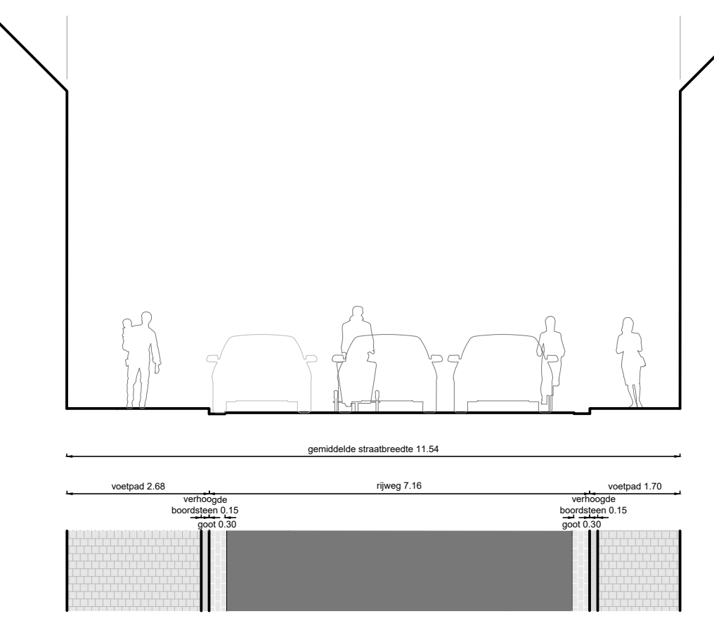
Dahliastraat typeprofiel breed - bestaand
