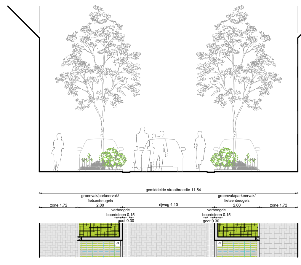
Dahliastraat typeprofiel breed - nieuw
