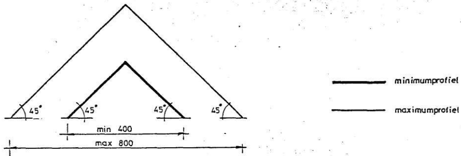
PROFIEL VAN DE SCHEIMUUR
