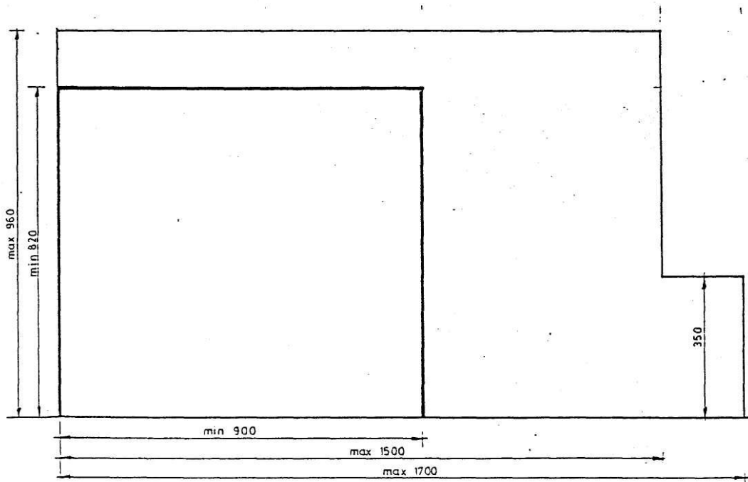
PROFIEL VAN DE SCHEIMUUR
