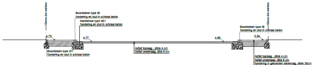
Snede B-B'
